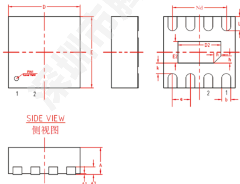
TOP VIEW 正视图
