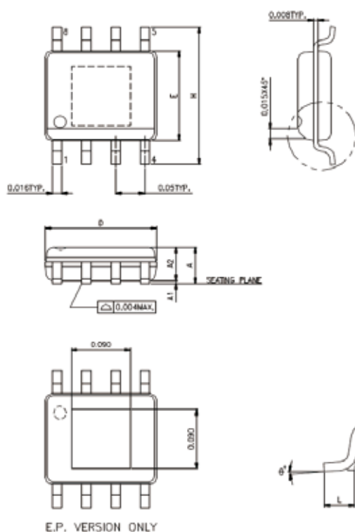
TOP VIEW 正视图
