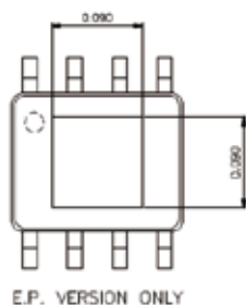
TOP VIEW 正视图
